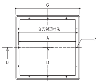
角型 ドーム伏図
