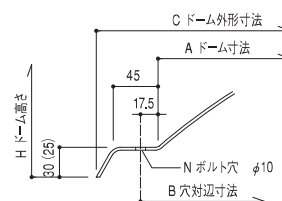
住宅用ドーム E 部詳細
