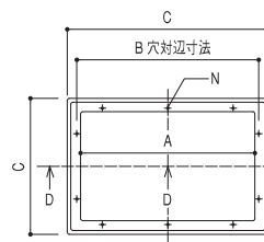
住宅用 ドーム伏図 P8 ホームトップライト用
