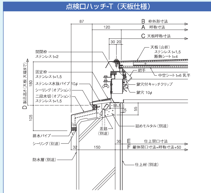
点検口ハッチ-T（天板仕様）
