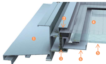
①固定枠 ②気密用パッキン ③断熱材 ④中空シート ⑤網入り型ガラス ⑥結露受け
