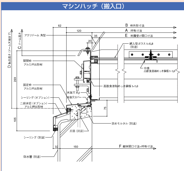
標準納まり図
